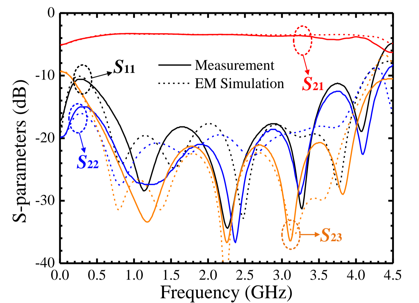
周波数特性
