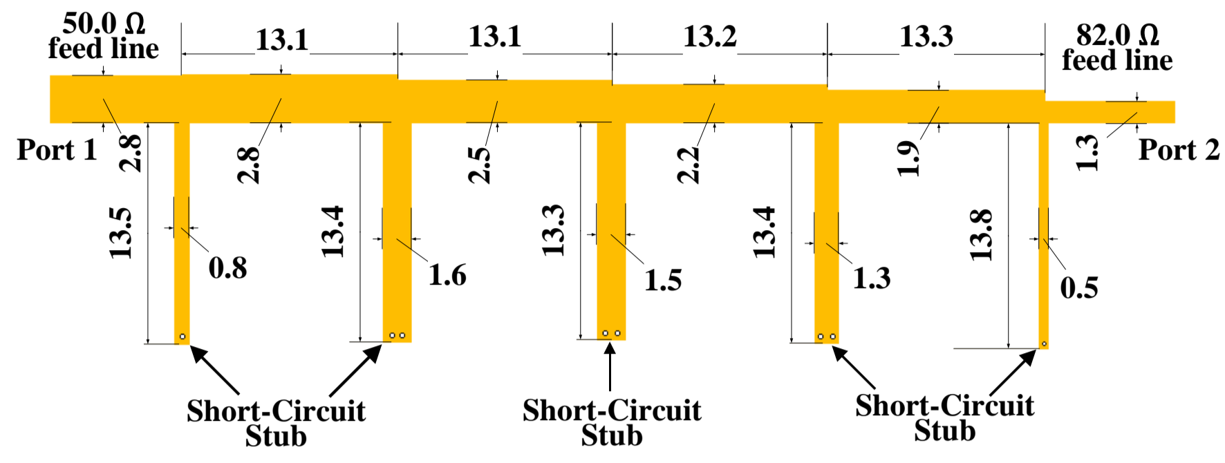
5段広帯域インピーダンス変成器 ( f_0=4 GHz, FBW=80\% , Z_S=50 \Omega , Z_L=82 \Omega )
