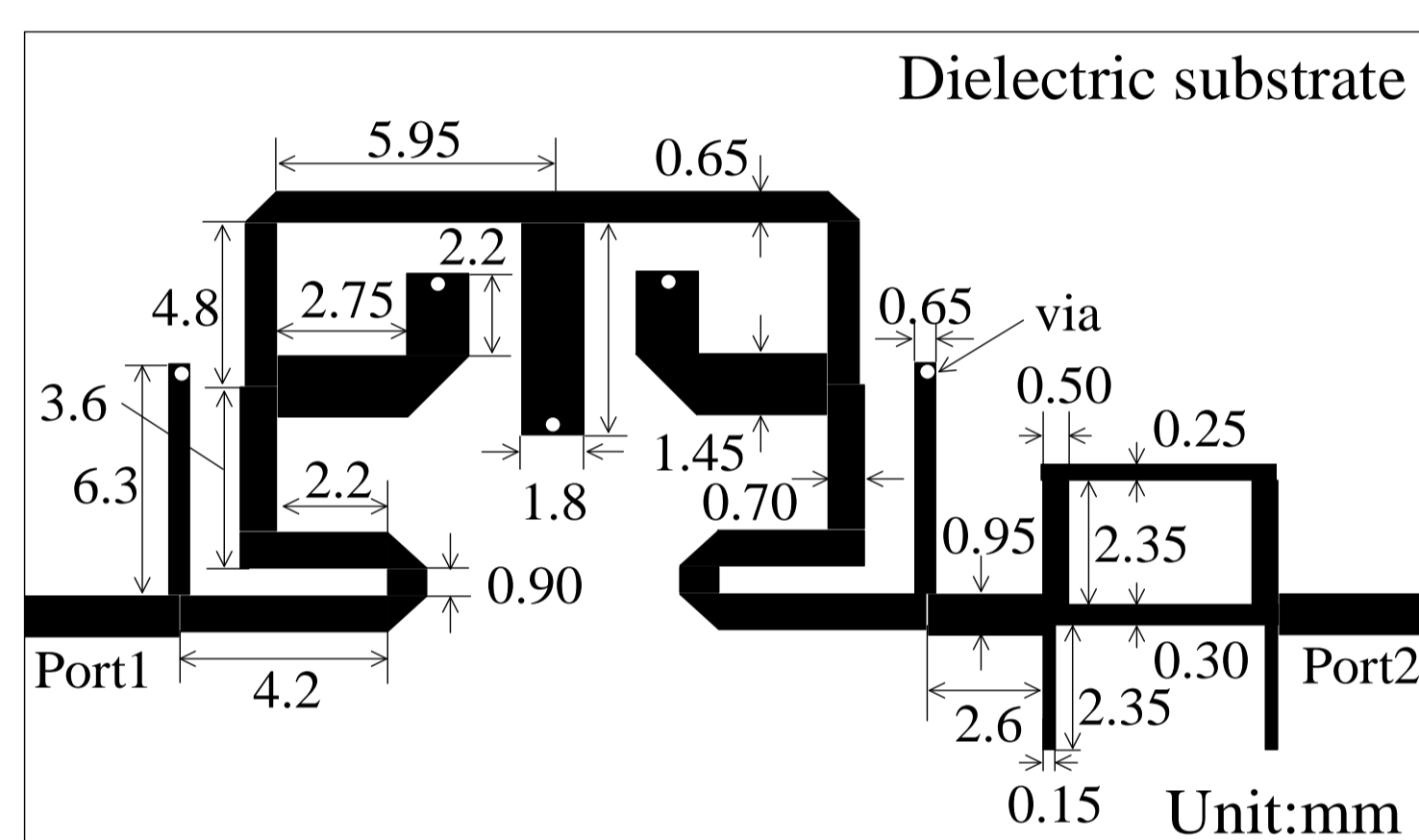
広い阻止域を有する9段階UWB BPF ( f_0=6.85 GHz, FBW=95\% )
