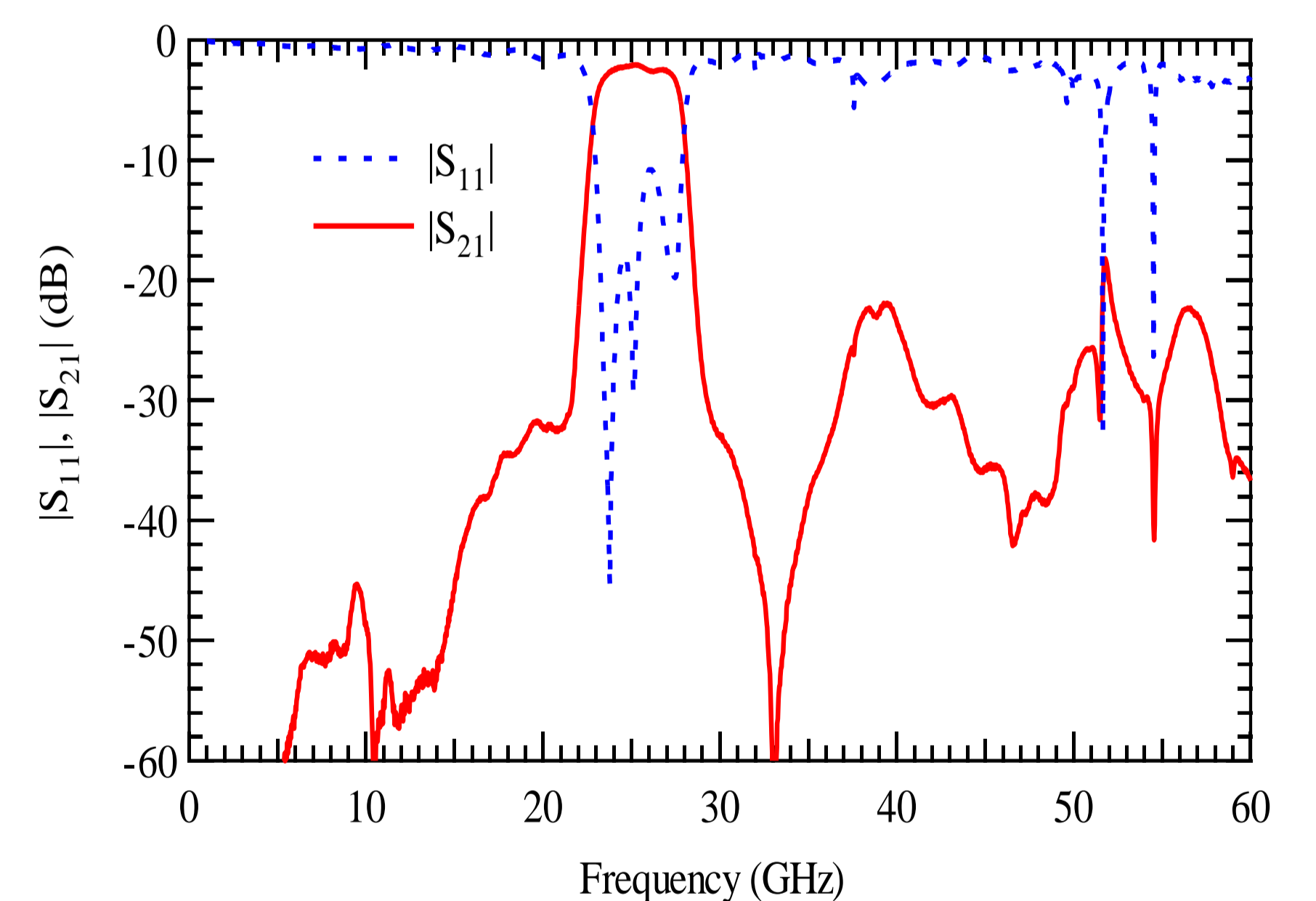
周波数特性
