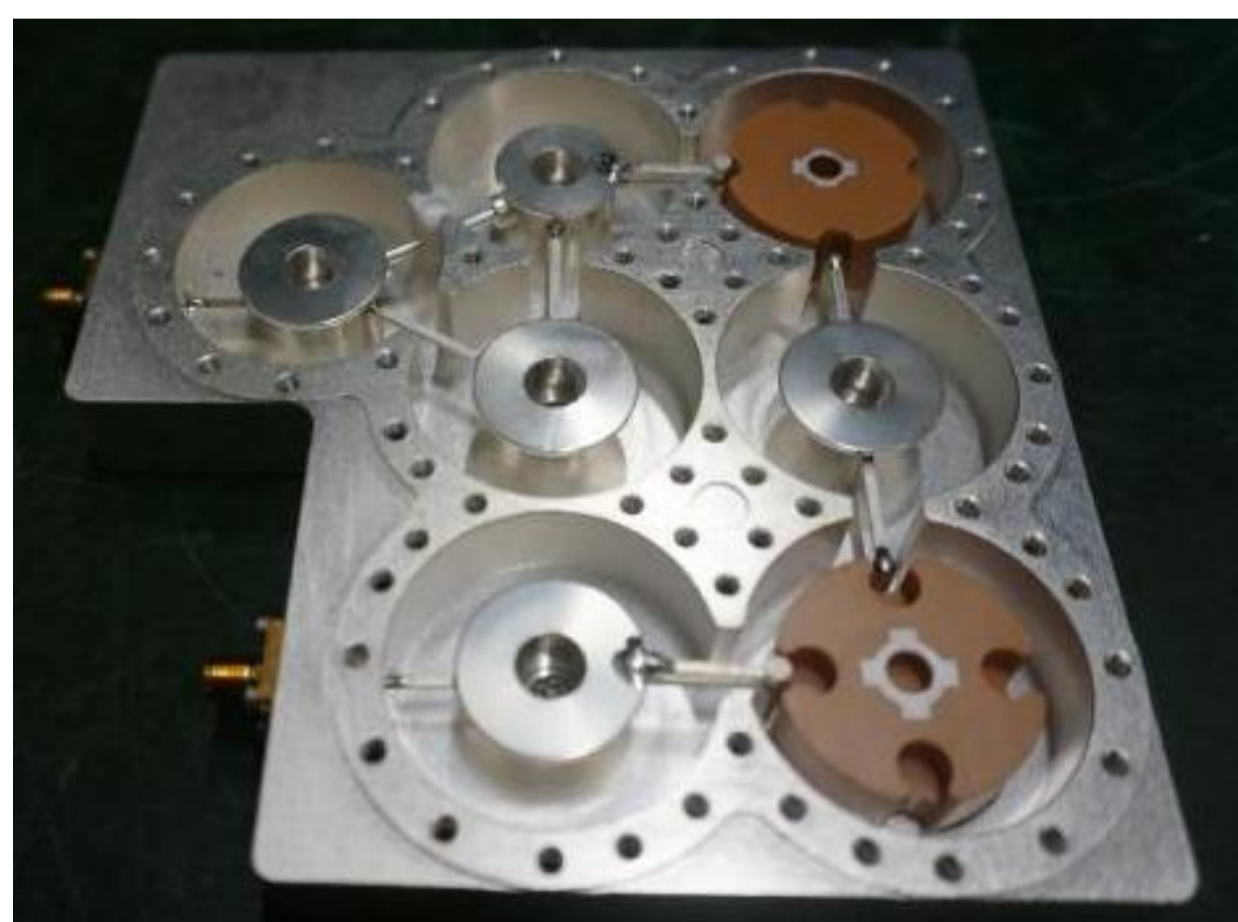
試作フィルタ
