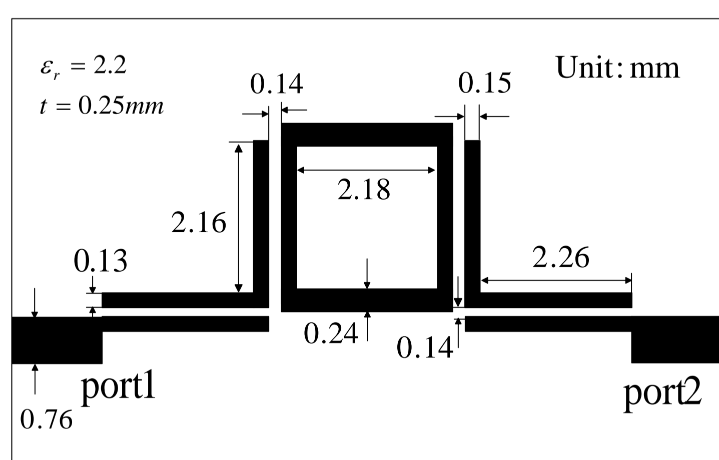
準ミリ波帯4段階UWB BPF ( f_0=25.5 GHz, 3dB- FBW=20\% )
