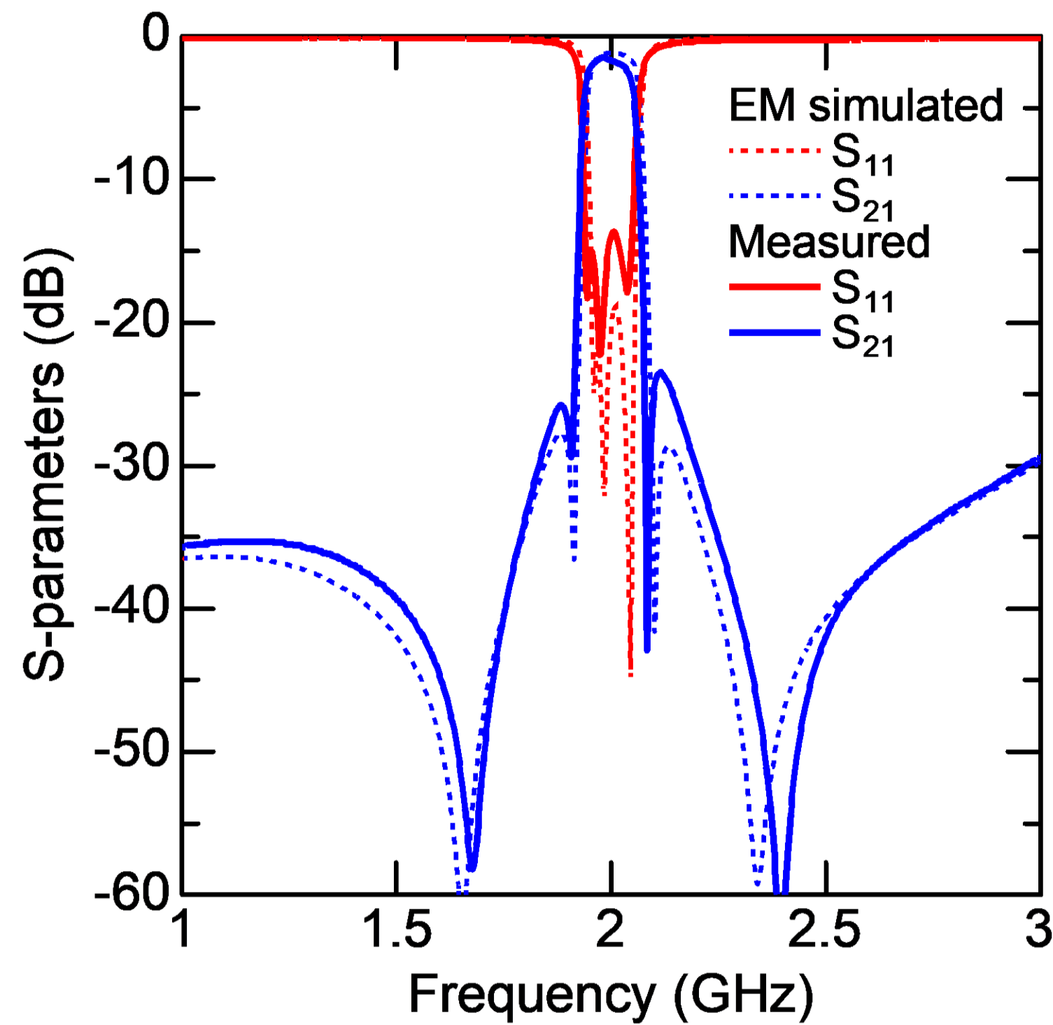
4 段Cul-de-Sac結合マイクロストリップBPF ( f_0=2 GHz, \Delta f=100 MHz)
