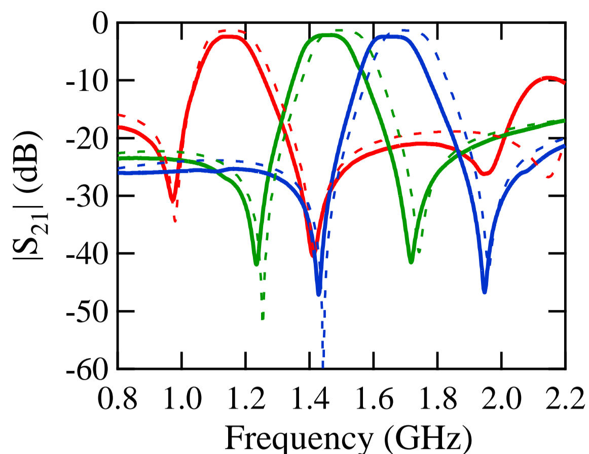
中心周波数可変
