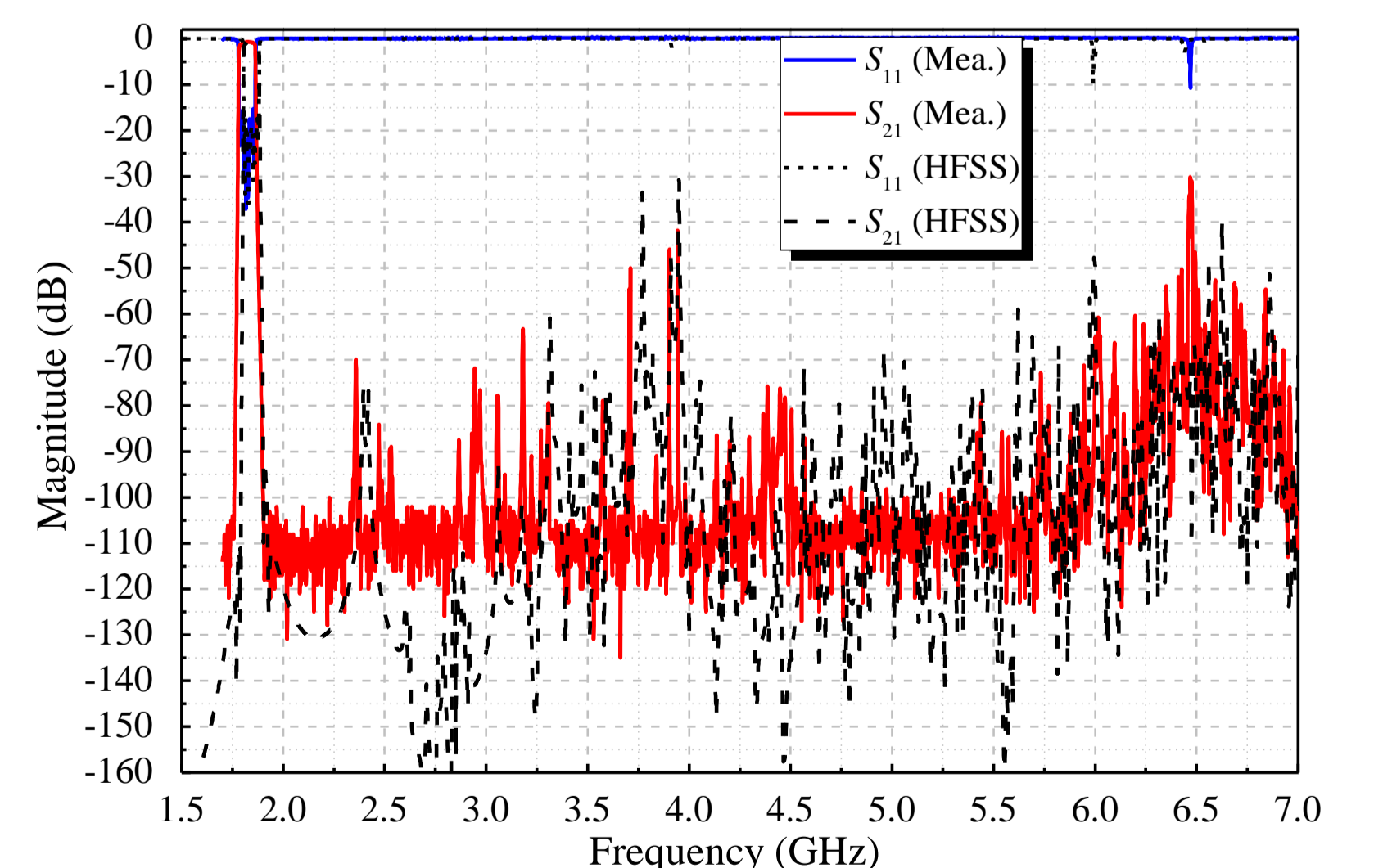
電磁界設計結果と測定結果
