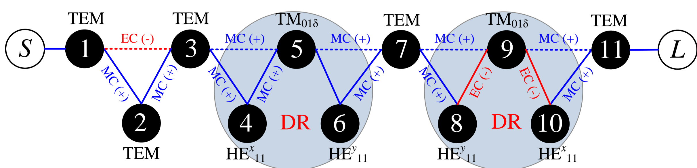
11段BPFの構成と結合トポロジー
