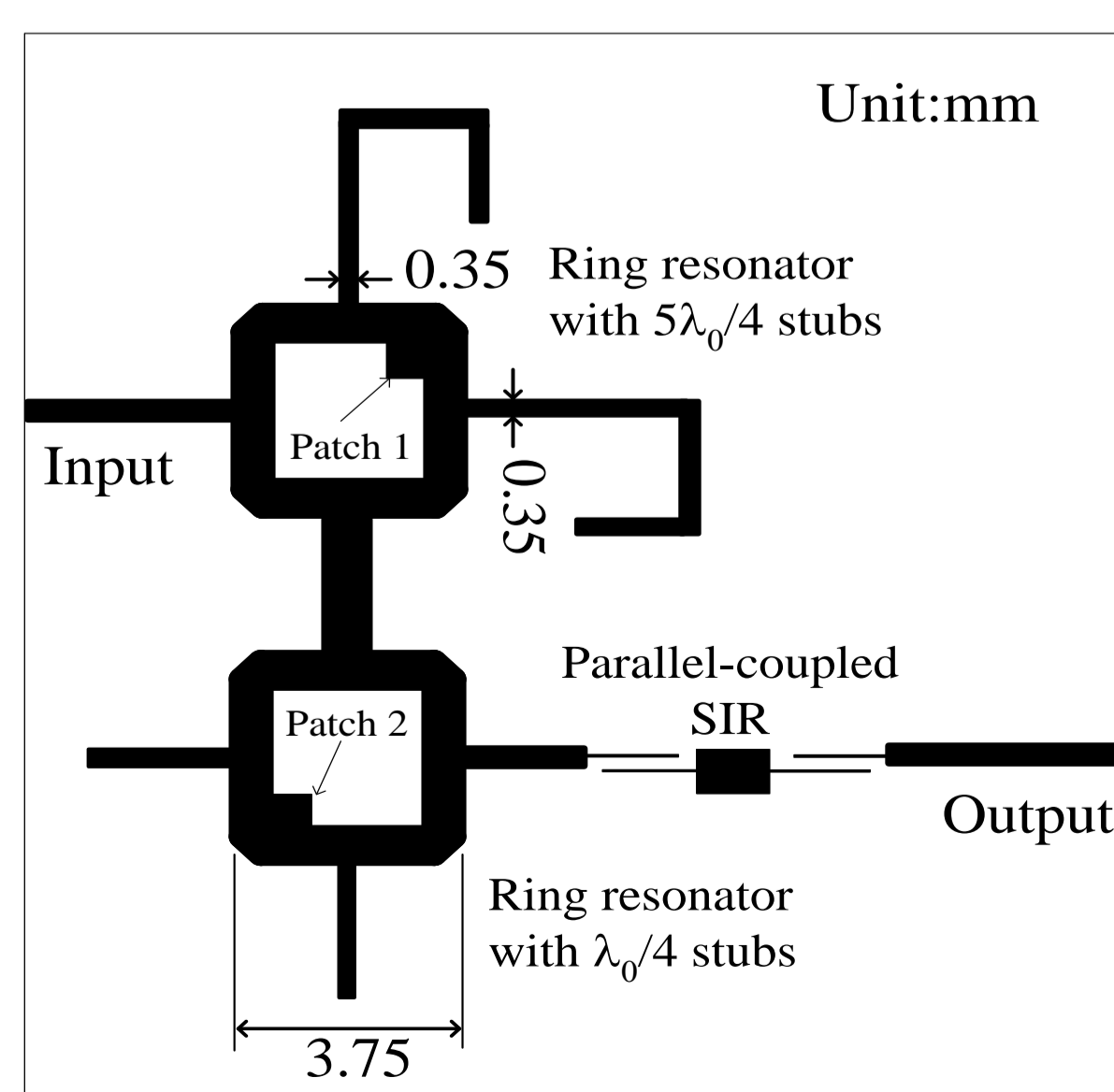
準ミリ波帯4段階UWB BPF ( f_0=25.5 GHz, 3dB- FBW=20\% )
