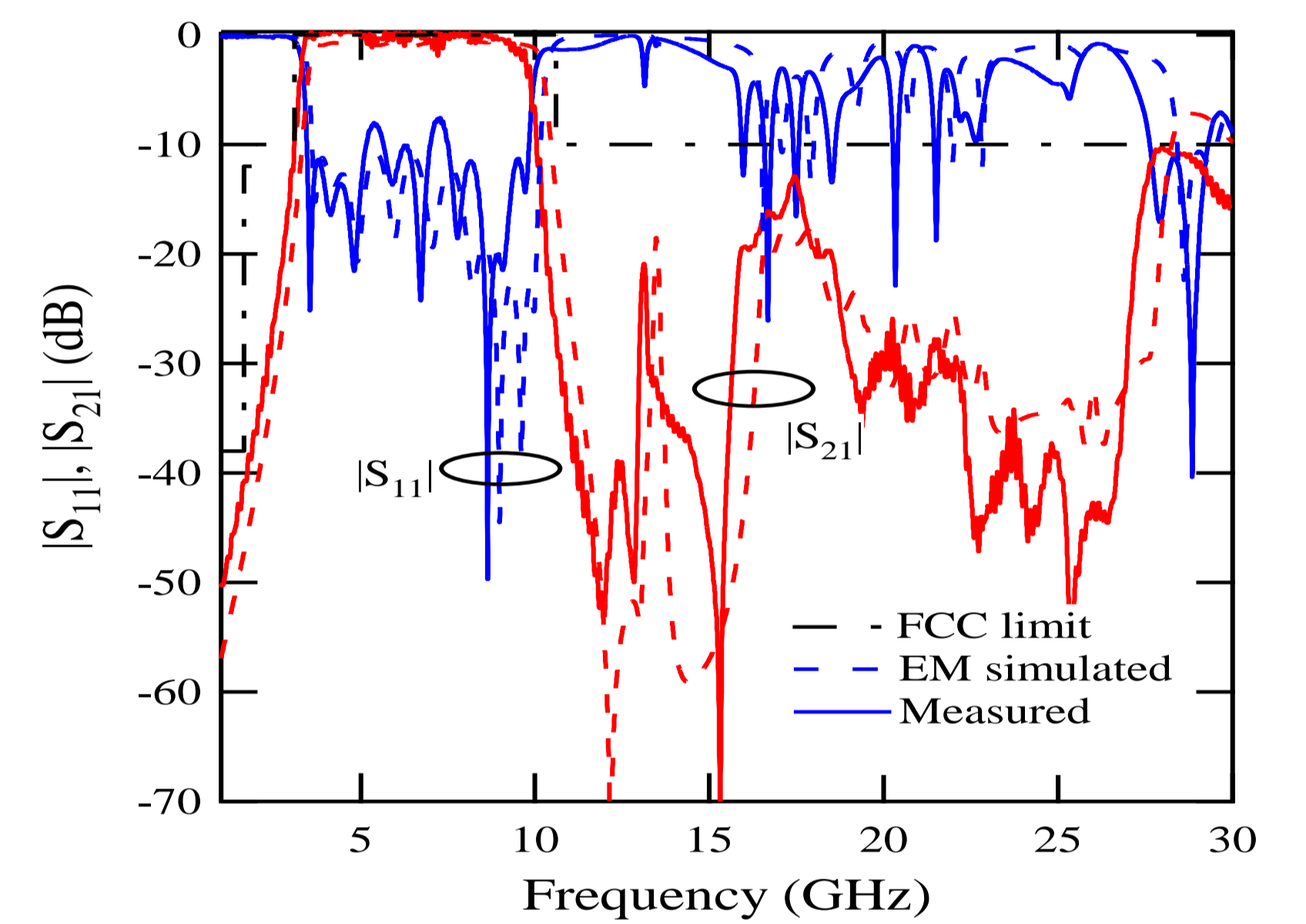
周波数特性
