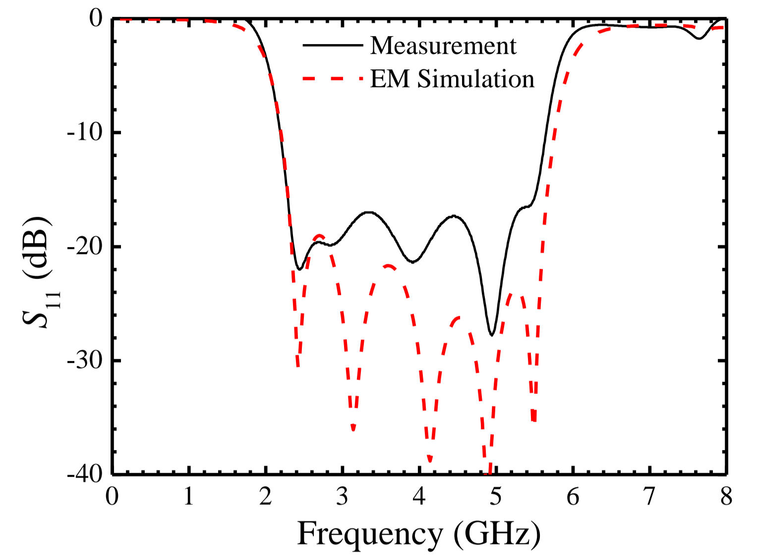
周波数特性
