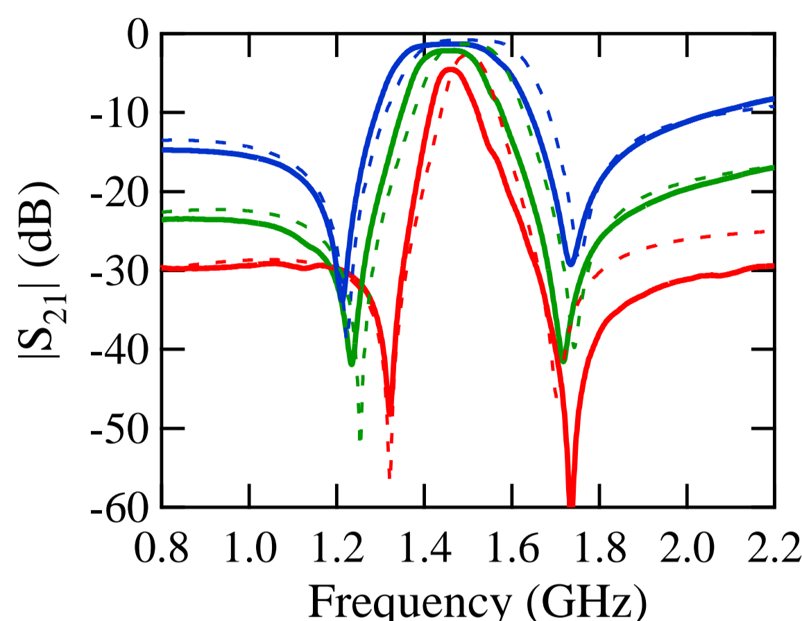
帯域幅可変
