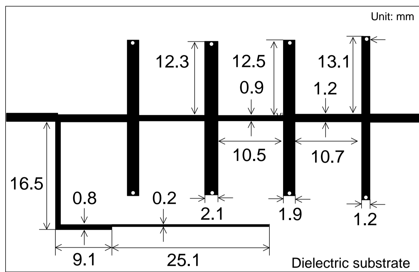
複数の伝送零点を有する5段階帯域BPF ( f_0=4 GHz, FBW=40\% )
