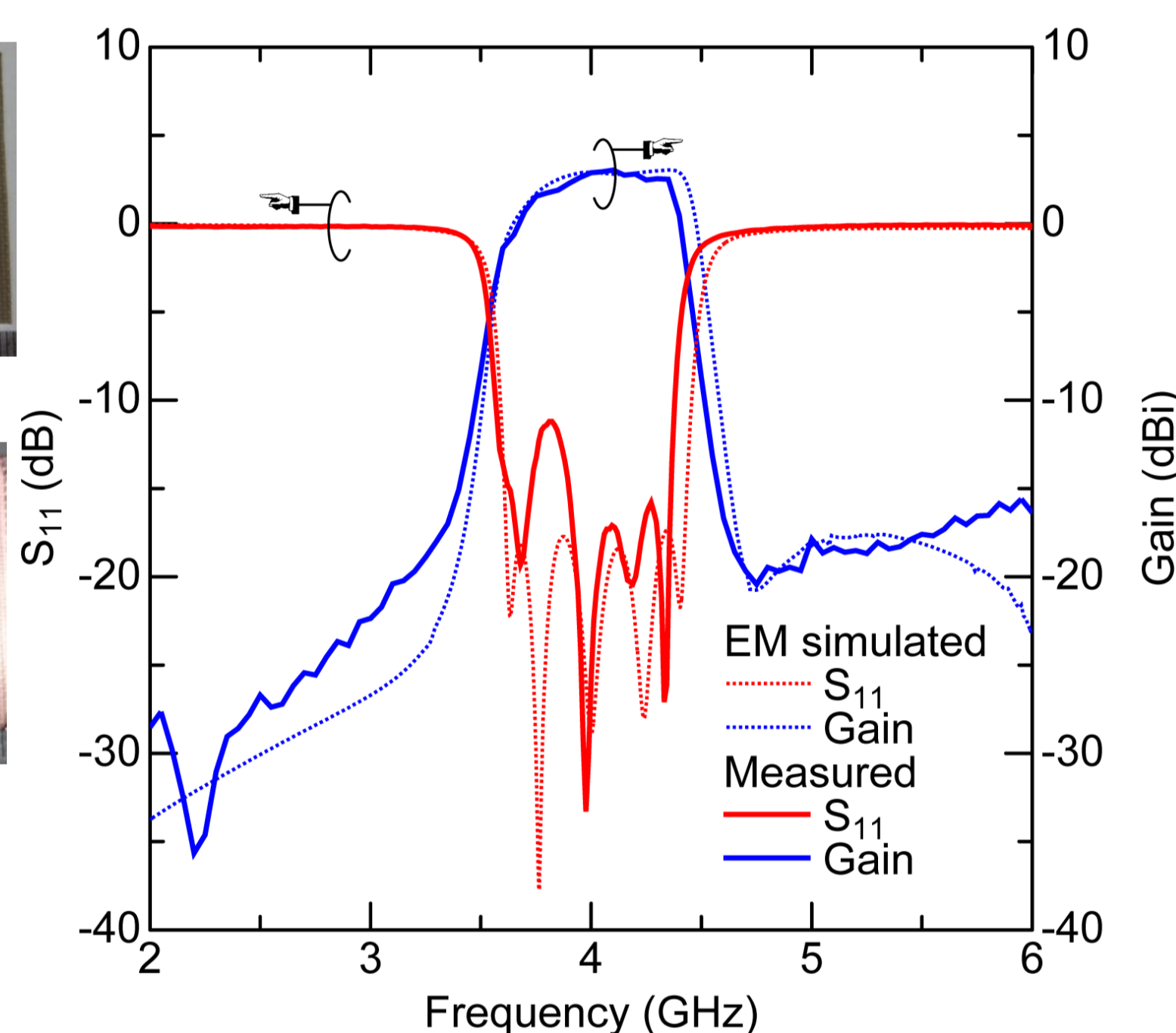
5段広帯域フィルテナ ( f_0=4.0\text{ GHz} , FBW=20\% )
