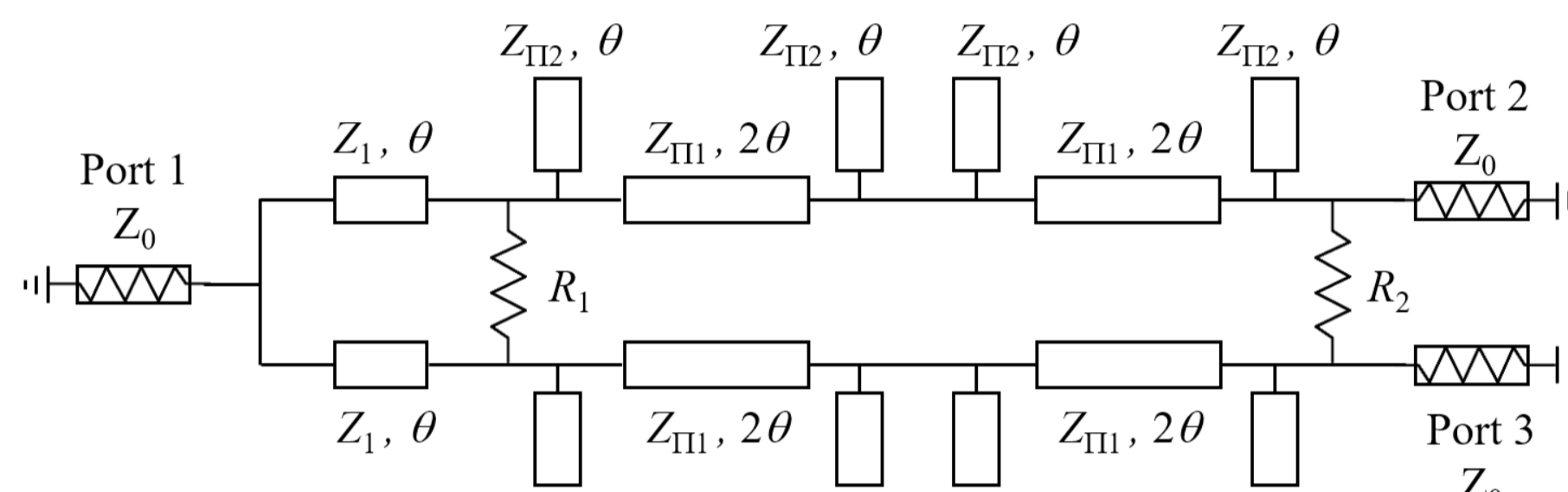
スタブ付き伝送線路を用いた提案電力分配器
