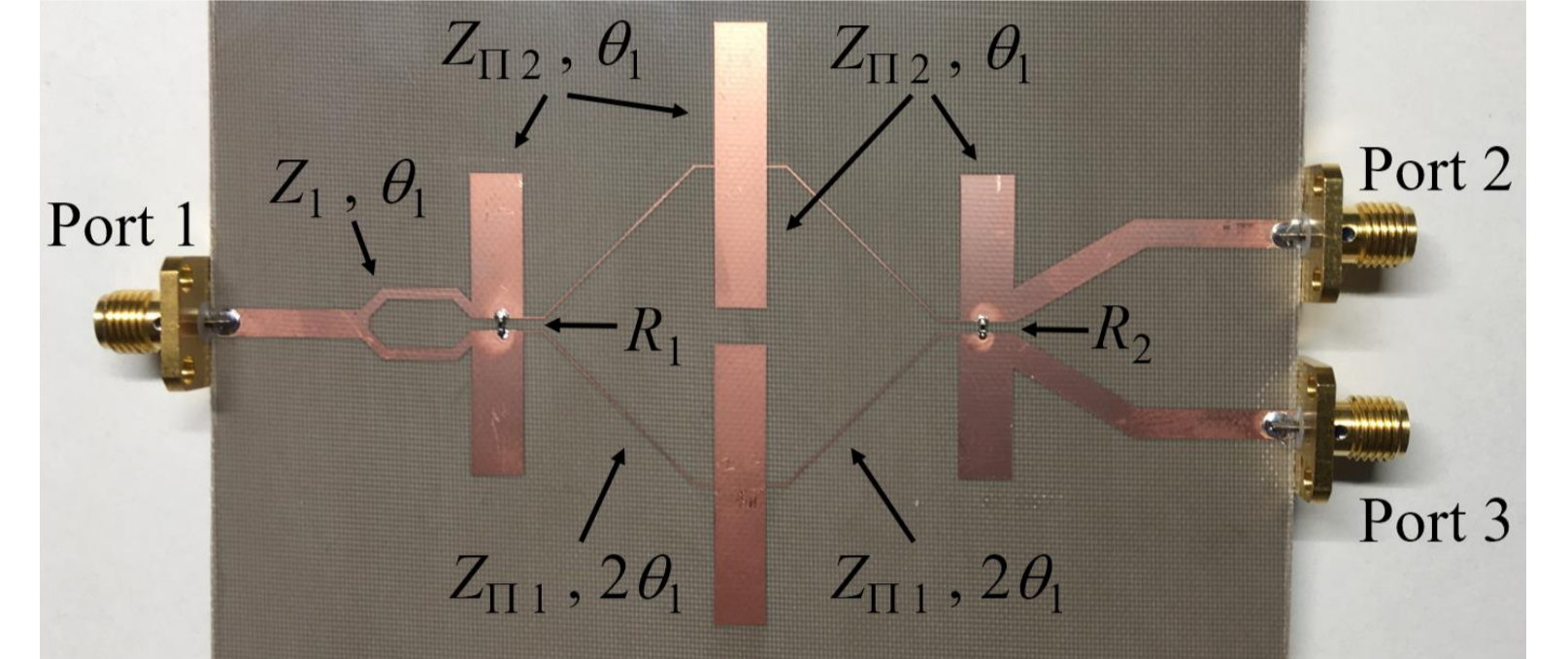
試作回路
