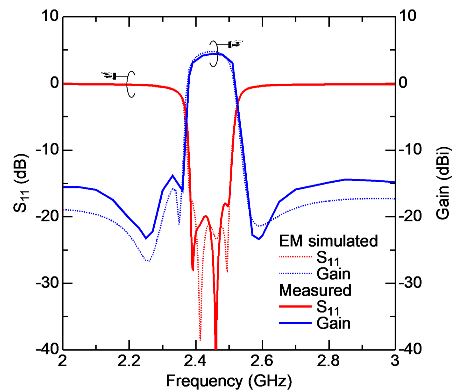
4段有極形狭帯域フィルテナ ( f_0=2.45\text{ GHz} , FBW=5\% )
