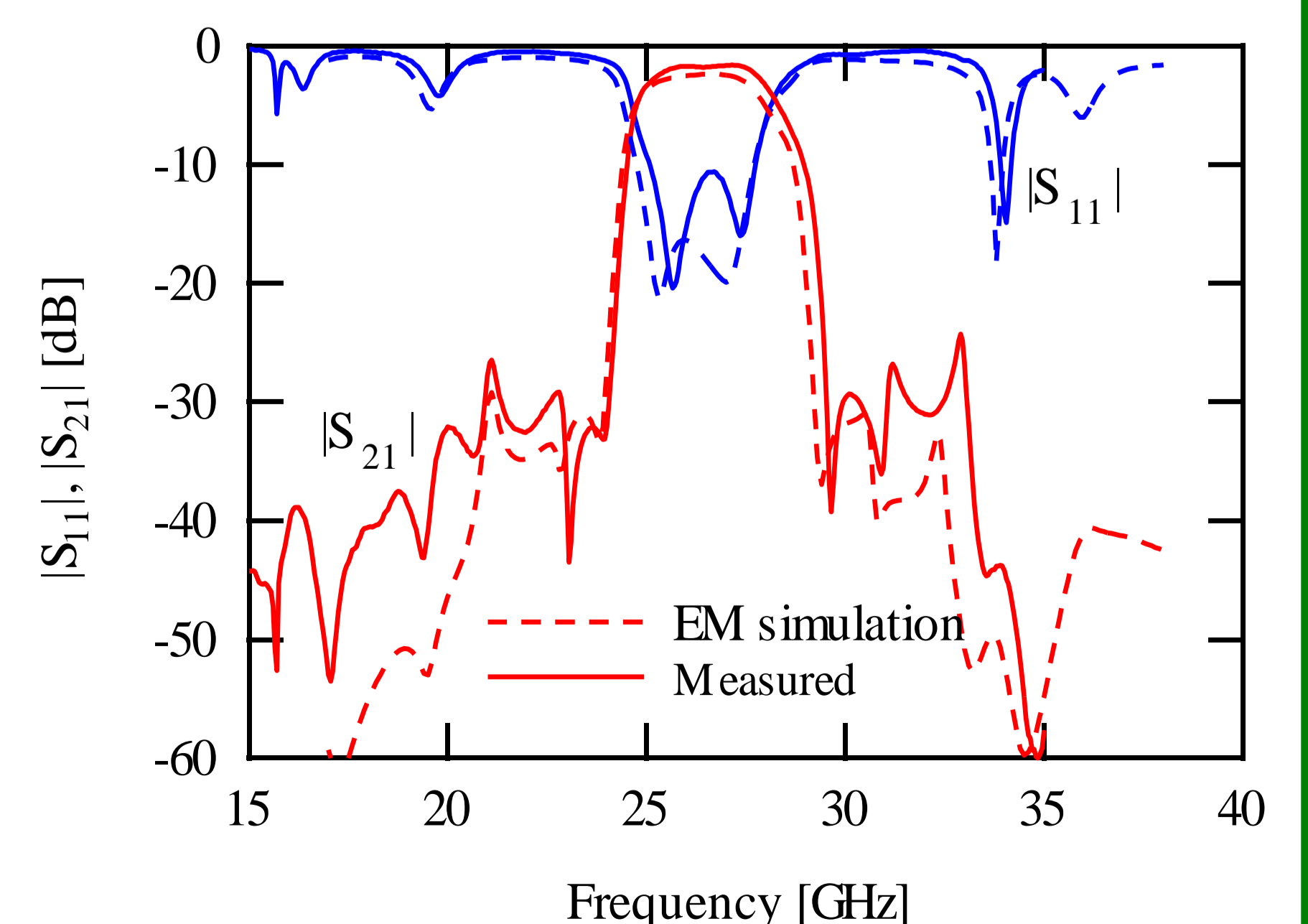
周波数特性
