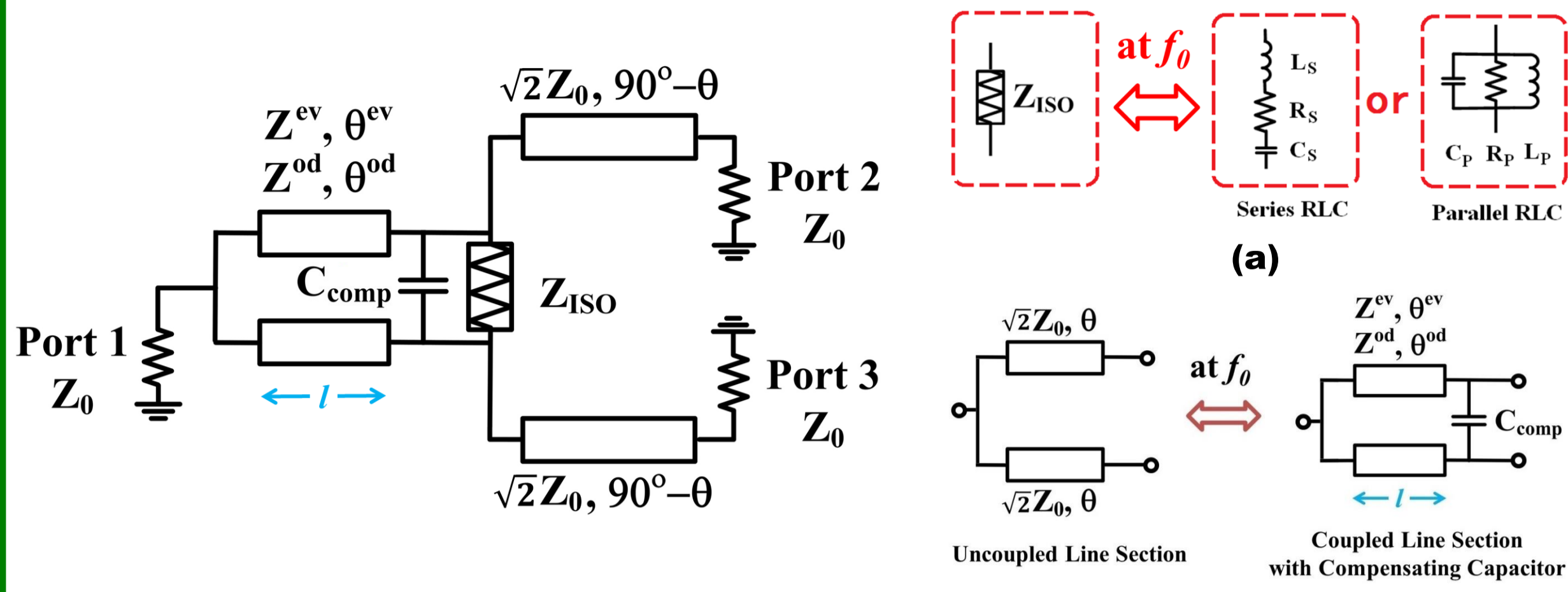
等価回路
