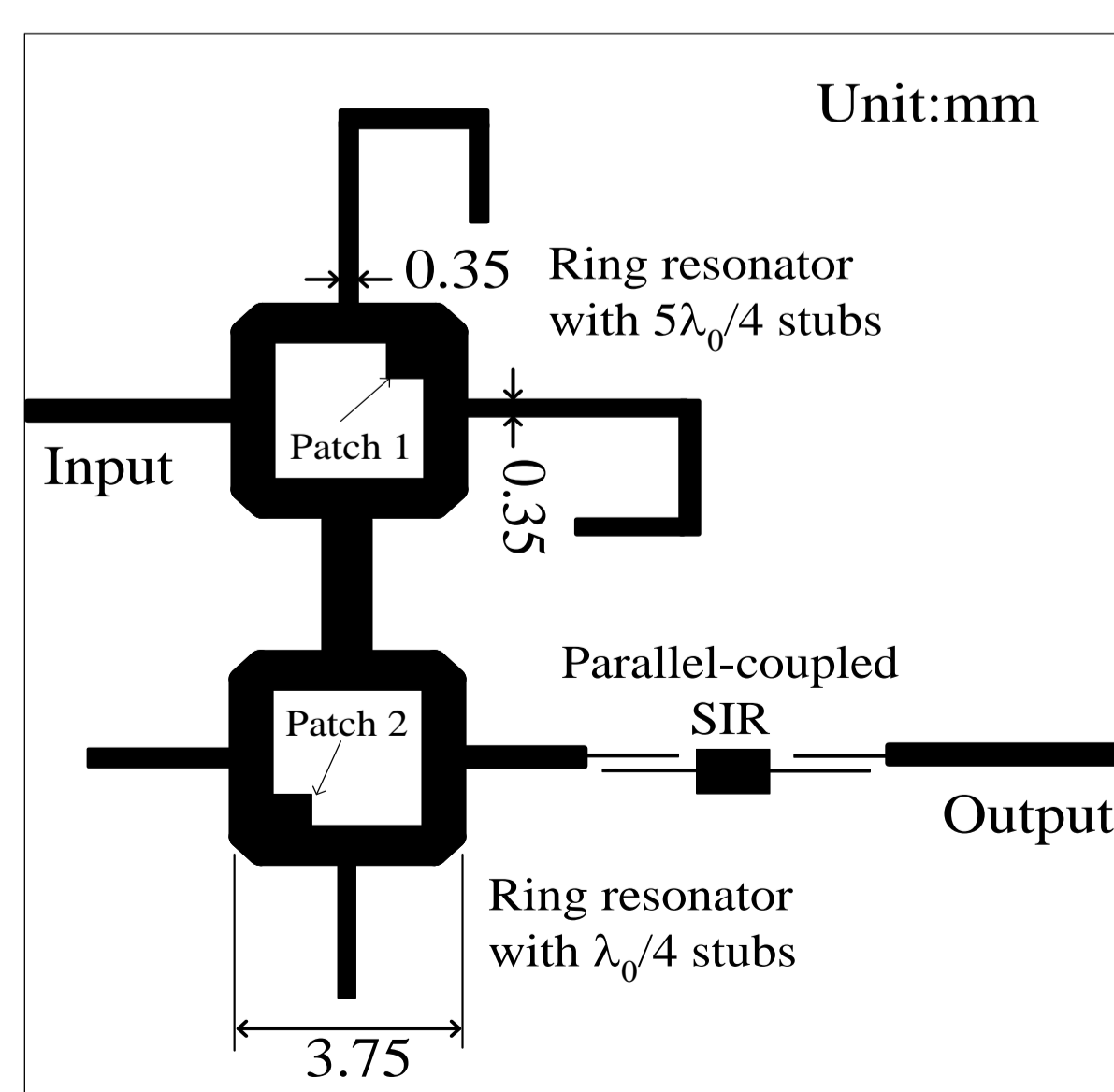
準ミリ波帯4段階UWB BPF ( f_0=25.5 GHz, 3\text{dB-}FBW=20\% )
