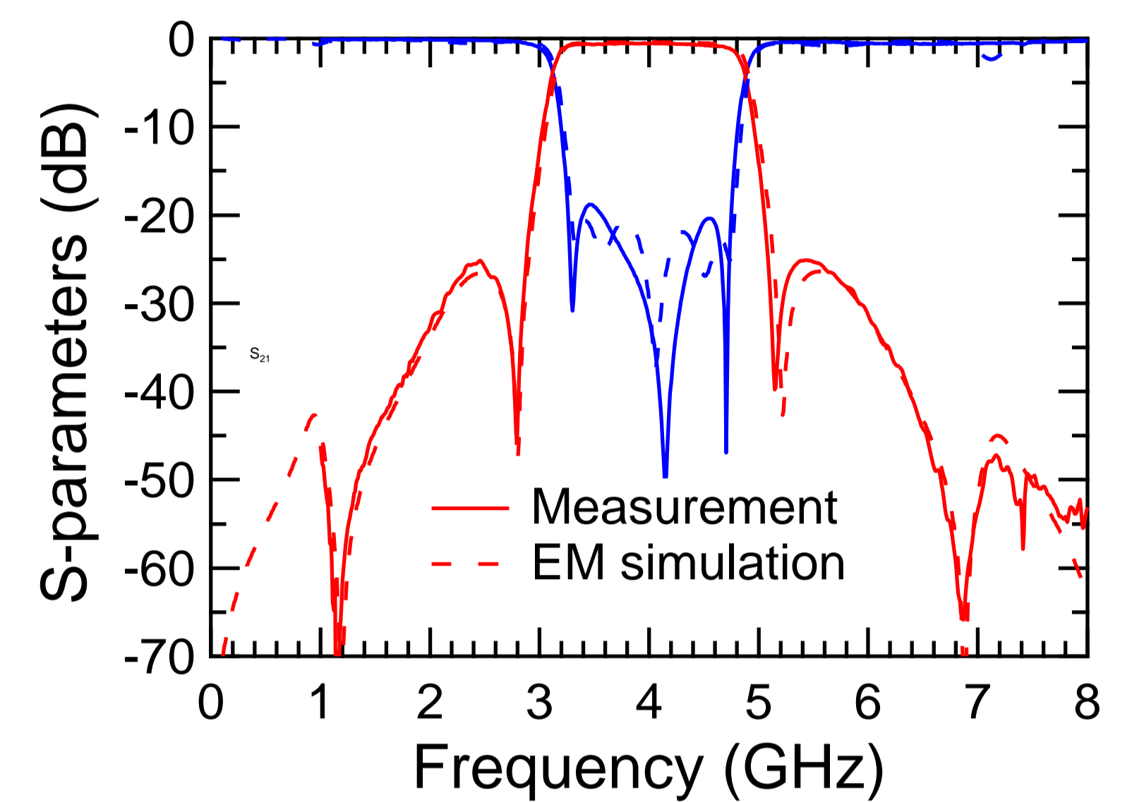
周波数特性
