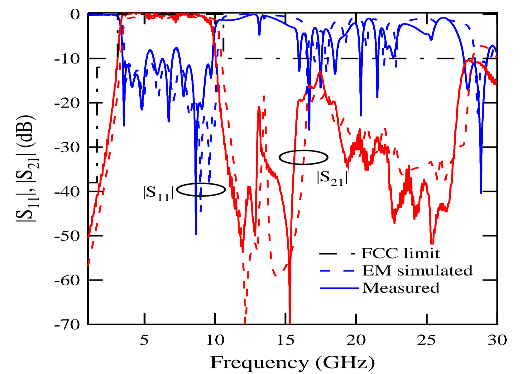
周波数特性
