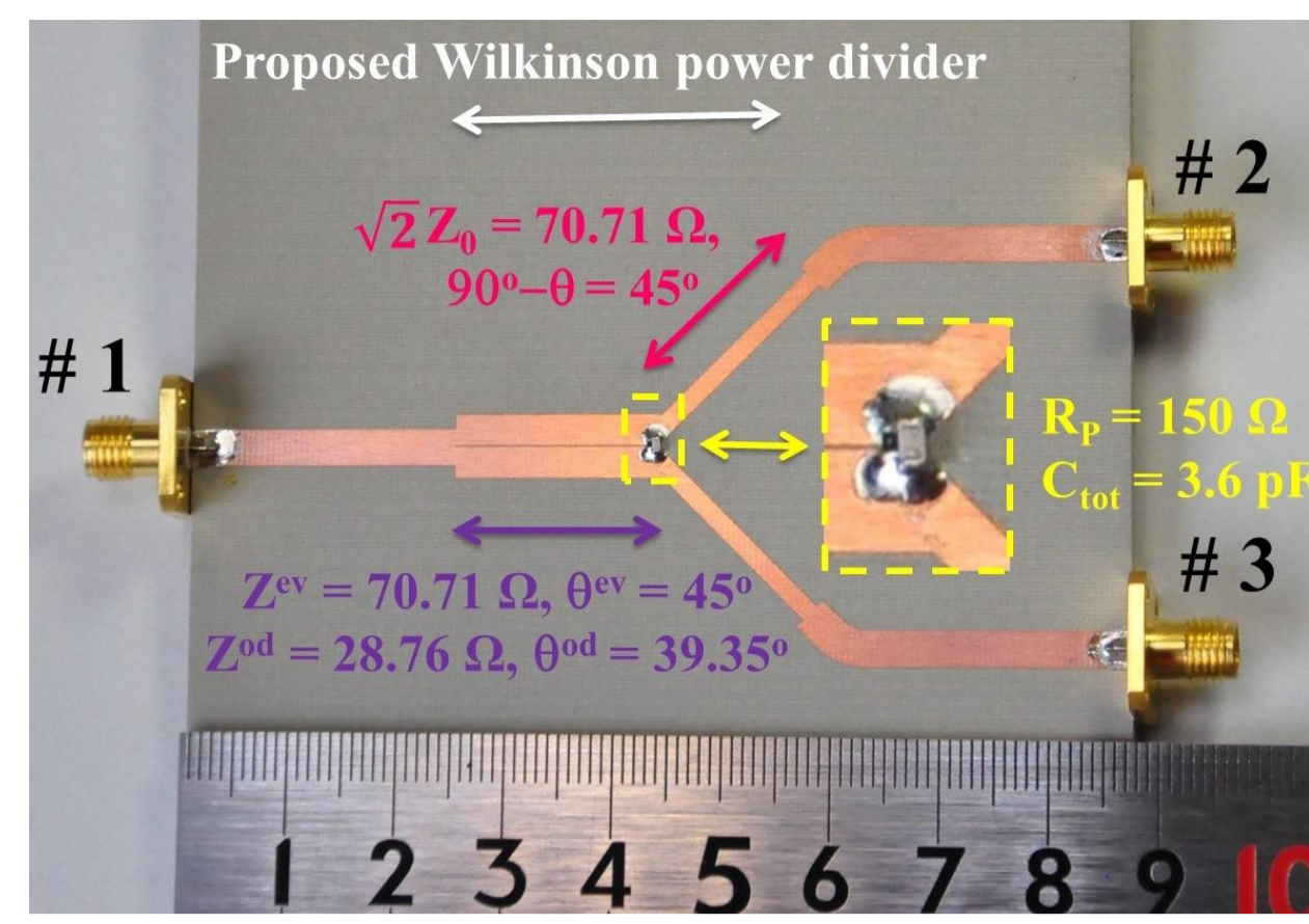
試作回路
