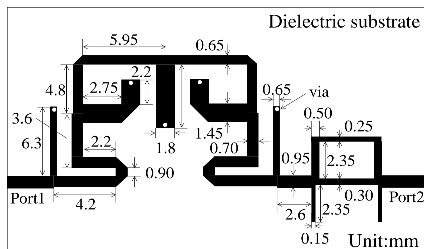
広い阻止域を有する9段階UWB BPF ( f_0=6.85 GHz, FBW=95\% )
