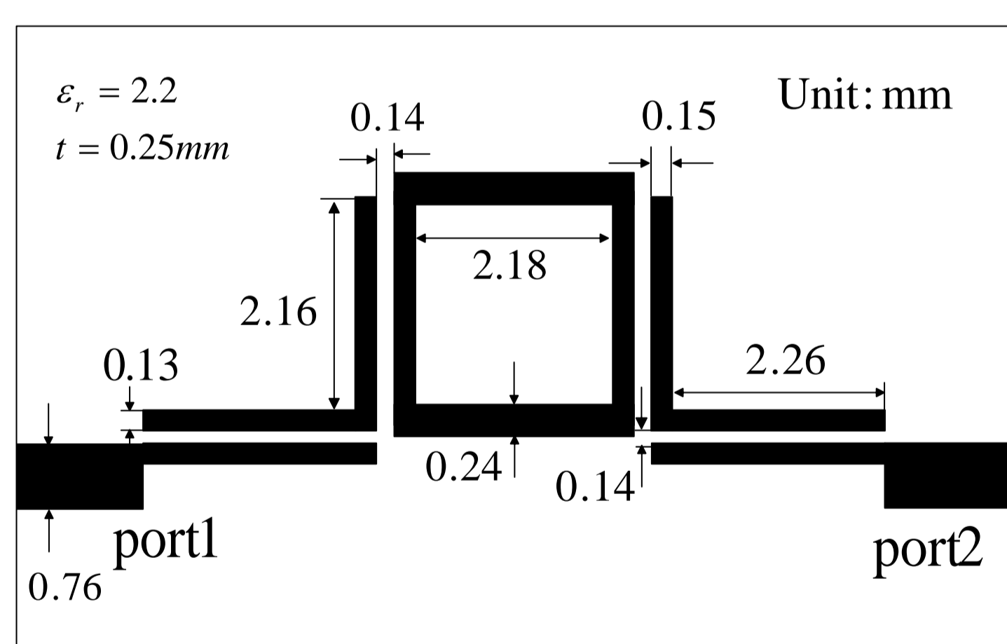
準ミリ波帯4段階UWB BPF ( f_0=25.5 GHz, 3\text{dB-}FBW=20\% )
