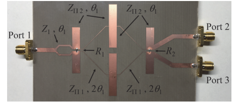
試作回路
