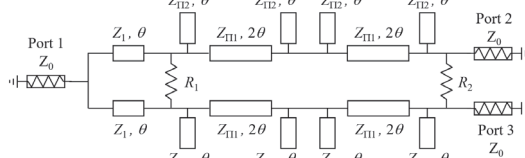
スタブ付き伝送線路を用いた 提案電力分配器
