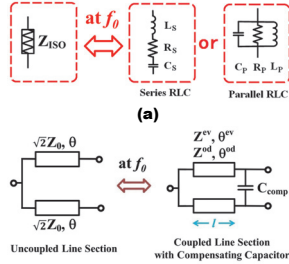
等価回路
