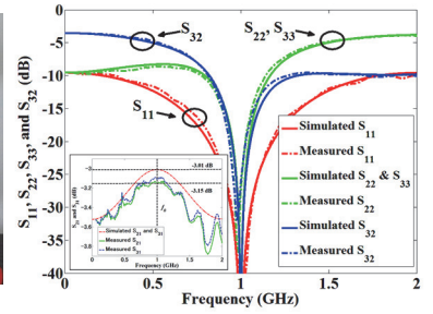
周波数特性
