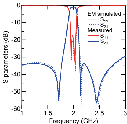
3段Cul-de-Sac結合フィルタ ( f_0=2\text{ GHz} , \Delta f=100\text{ MHz} )
