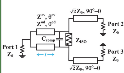
提案電力分配器
