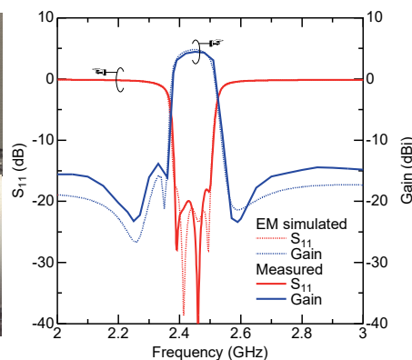
4段有極形フィルテナ ( f_0=2.45\text{ GHz} , FBW=5\% )
