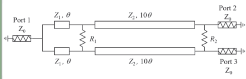
提案デュアルバンド電力分配器
