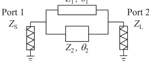
提案する並列型伝送線路変成器 (デュアルバンド)
